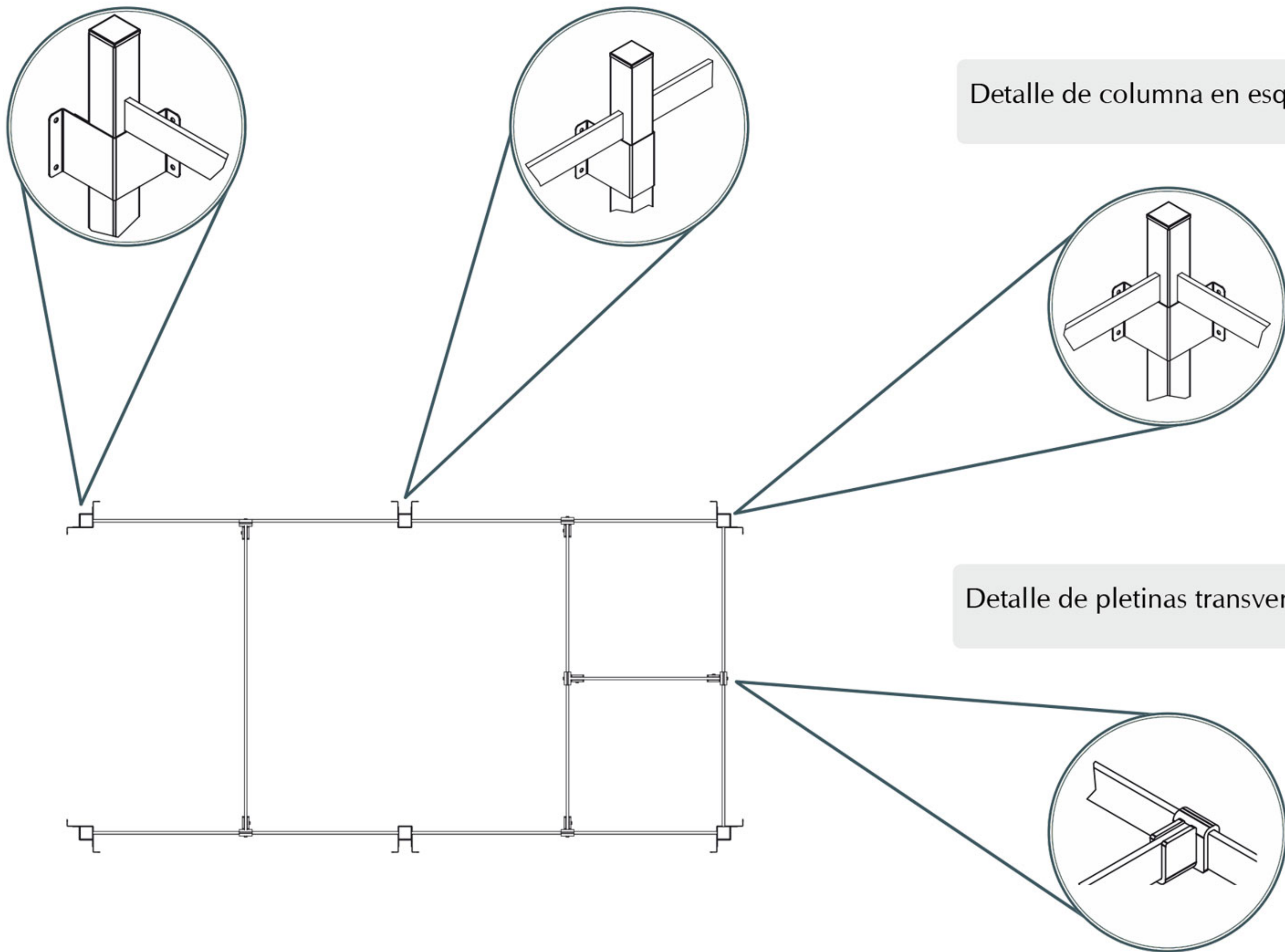
Detalle de columna terminal.
