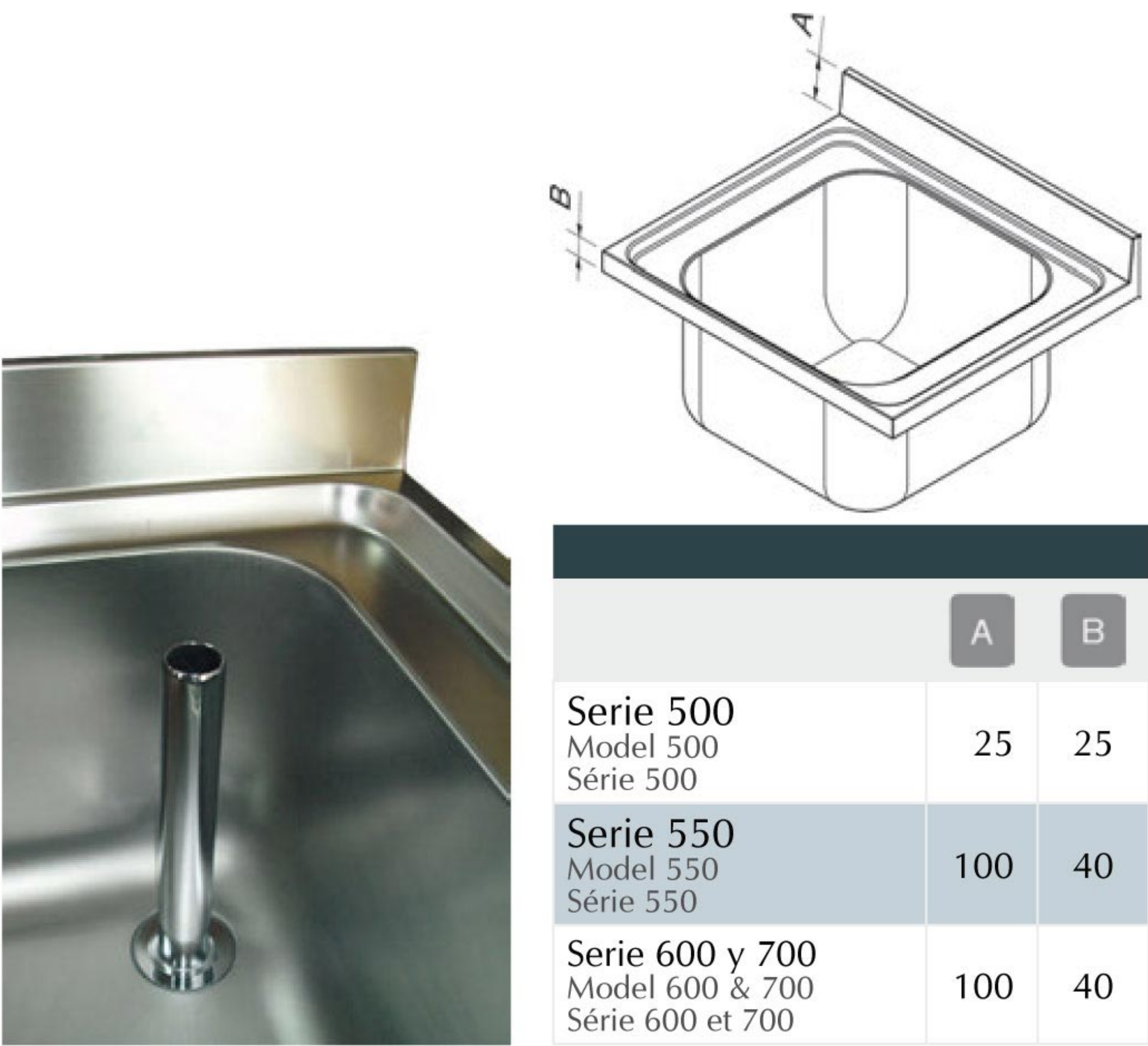
Detalle de tubo rebosadero (Fregaderos de ancho 600 y 700 mm ) Overflow detail. (600 y 700 mm sinks) Détail de tube-déversoir (profondeur 600 et 700 mm)
