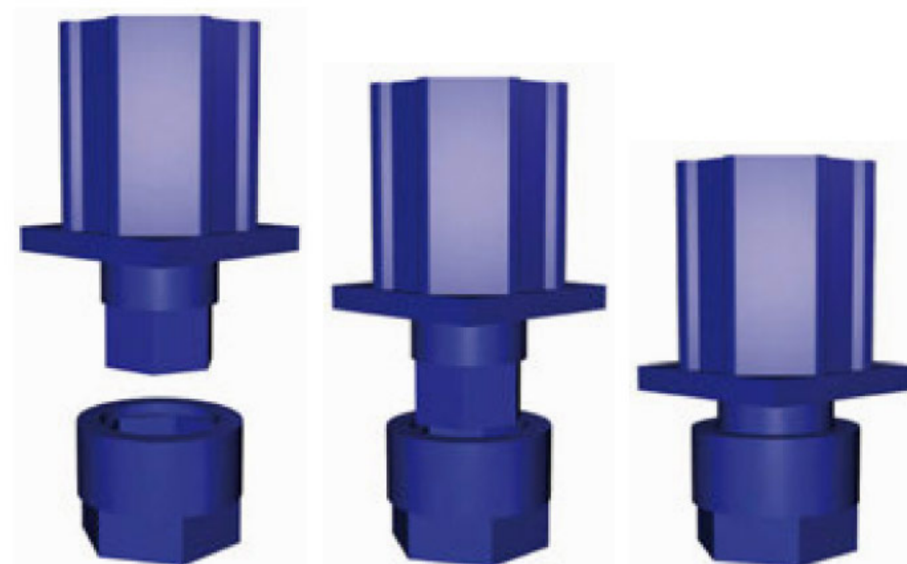
Detalle de pata con pie regulable con funda antivibradora.
